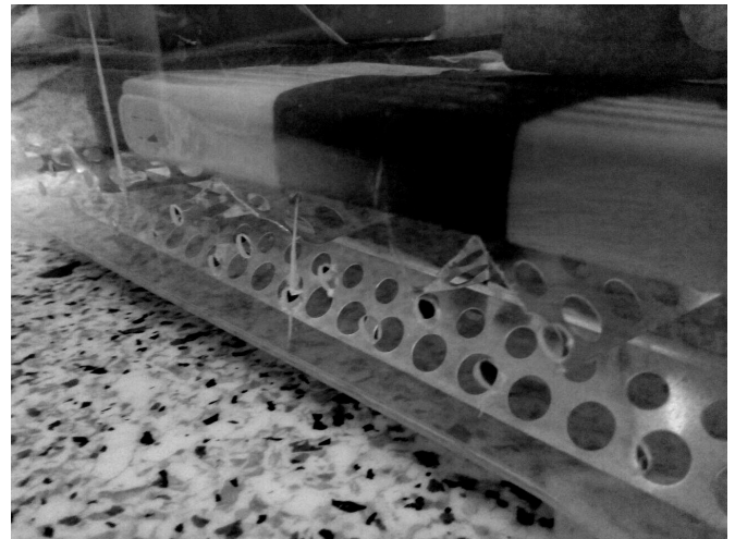
Abbildung 2. Ansauglöcher und Aluprofile
